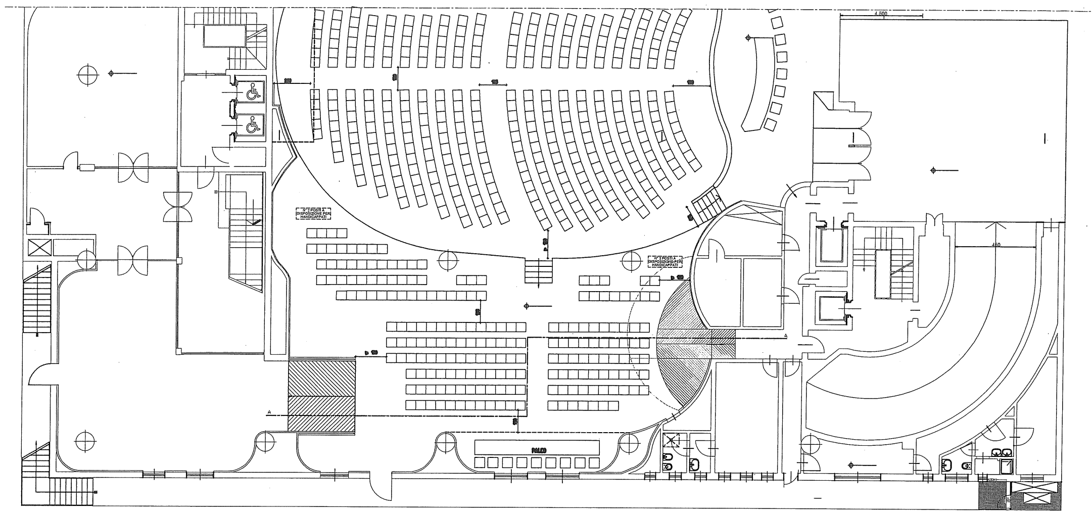
SEZIONE A-A
